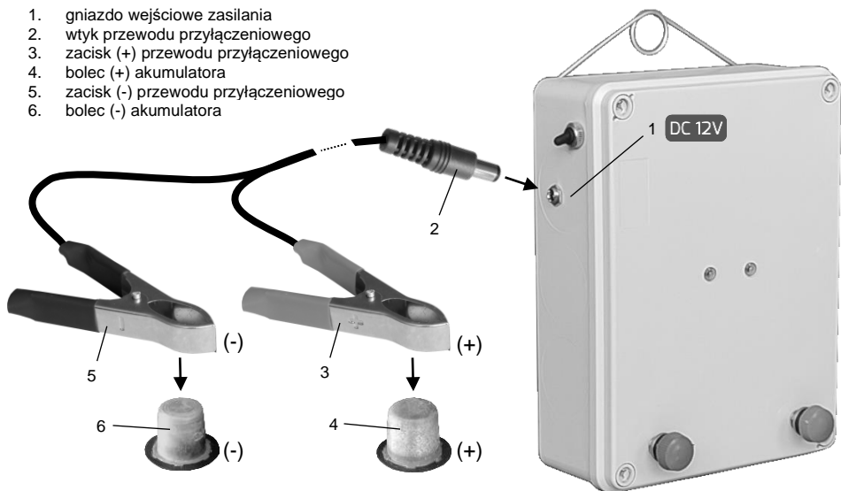
Rys. 2. Sposób przyłączenia elektryzatora do akumulatora.
