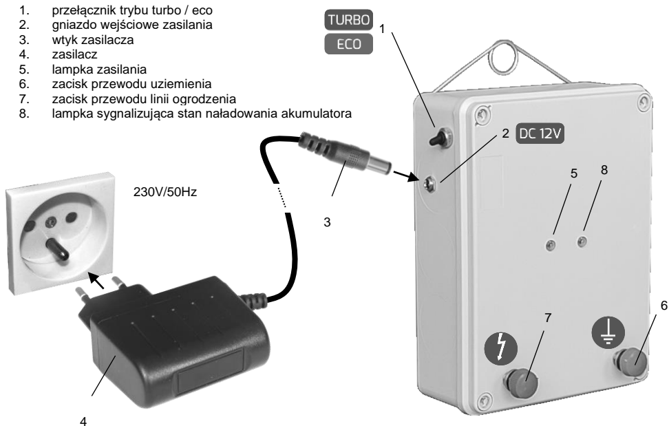
Rys. 1. Opis elektryzatora i sposób podłączenia zasilania z sieci elektrycznej ~230V
