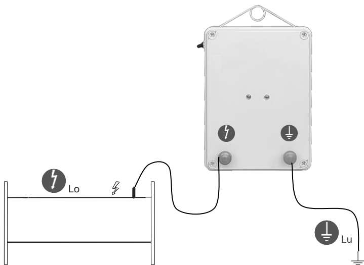
Rys. 3. Sposób przyłączenia elektryzatora do linii ogrodzenia (Lo) i linii uziemienia (Lu)
