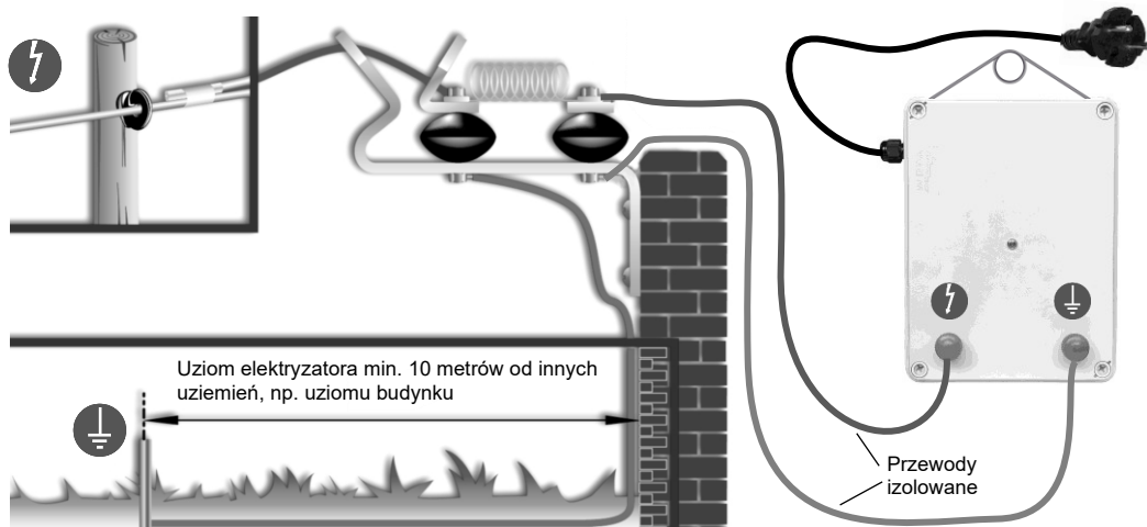
Rys. nr 3 - Przykładowe zainstalowanie odgromnika, oraz jego prawidłowe podłączenie do elektryzatora i uziomu.
