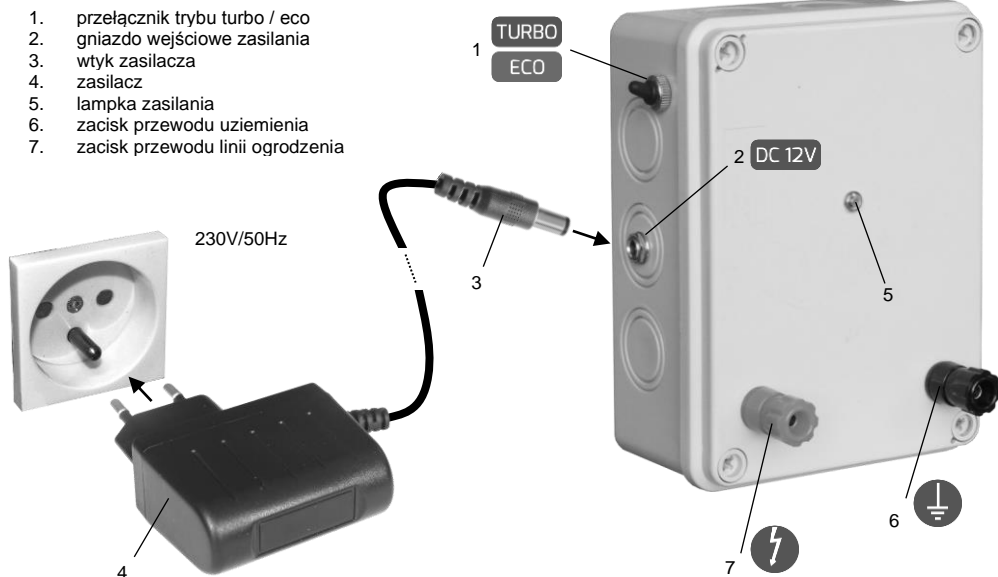
Rys. 1. Opis elektryzatora i sposób podłączenia zasilania z sieci elektrycznej ~230V
