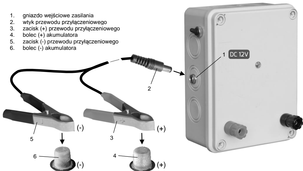
Rys. 2. Sposób przyłączenia elektryzatora do akumulatora.
