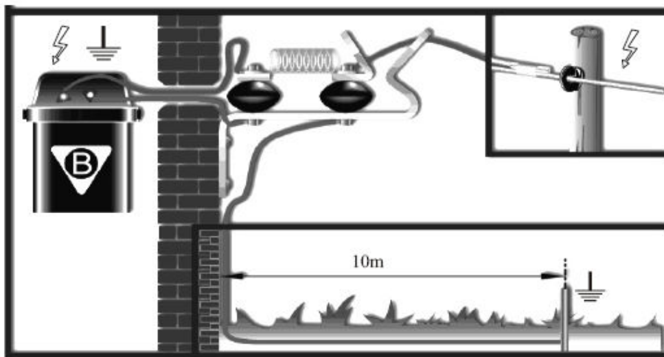
Rys. 4 Sposób przyłączenia odgromnika
