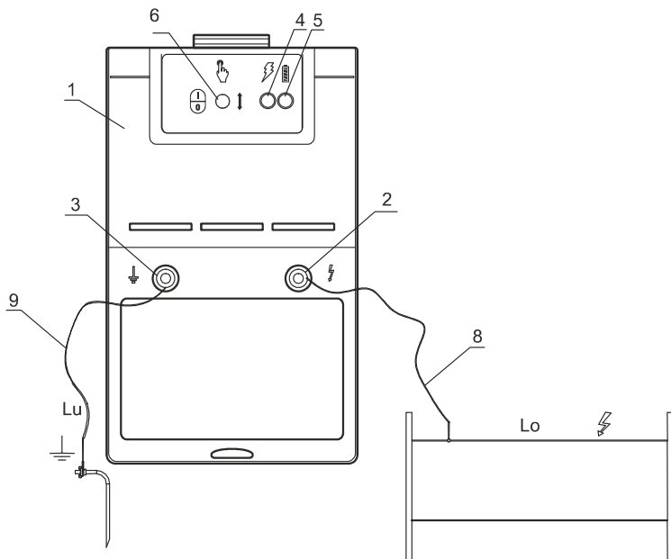
Rys. 1. Podłączenie zasilania z sieci elektrycznej ~230V
