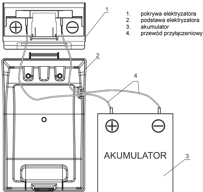
Rys. 3. Sposób przyłączenia elektryzatora GATOR 500+ do akumulatora
