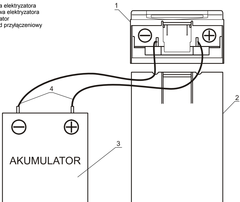
Rys. 3. Sposób przyłączenia elektryzatora ECOSTOP do akumulatora.
