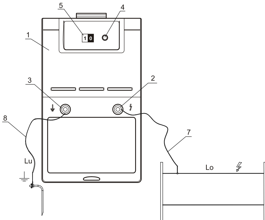
Rys. 2. Części składowe i sposób przyłączenia elektryzatora ECOSTOP do zasilacza AC 12V/150mA, linii ogrodzenia /Lo/ i linii uziemienia /Lu/
