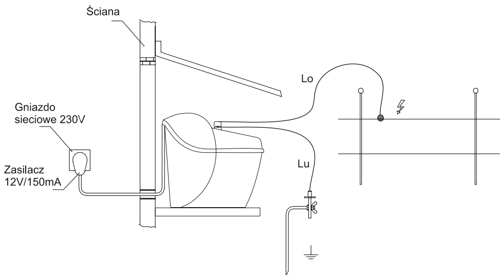
Rys. 4. Sposób instalowania elektryzatora ECOSTOP zasilanego z sieci poprzez zasilacz AC 12V/150mA. /Lu/ - linia uziemienia, /Lo/ - linia ogrodzenia
