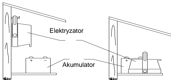
Rys. 6 Sposób instalowania elektryzatora EBS-872/M zasilanego z akumulatora
