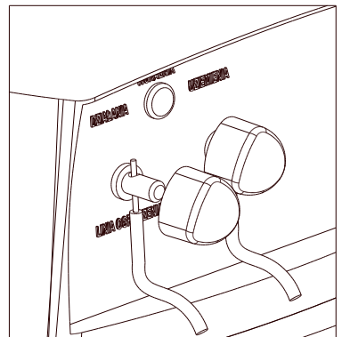
Rys. 2 Części składowe i sposób podłączenia elektryzatora EBS-872/M do zasilacza AC 12V/1000mA, linii ogrodzenia /Lo/ i linii uziemienia /Lu/
