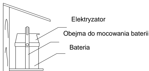
Rys. 5 Sposób instalowania elektryzatora EBS-872/M zasilanego z baterii
