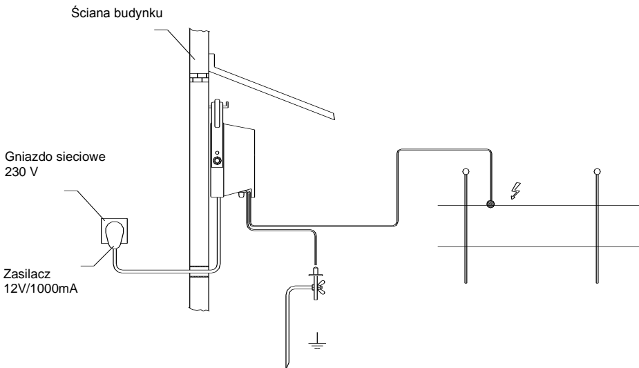
Rys. 3. Sposób instalowania i podłączenia elektryzatora EBS-872/M zasilanego z sieci poprzez zasilacz AC 12V/1000mA. /Lu - linia uziemienia, Lo - linia ogrodzenia/
