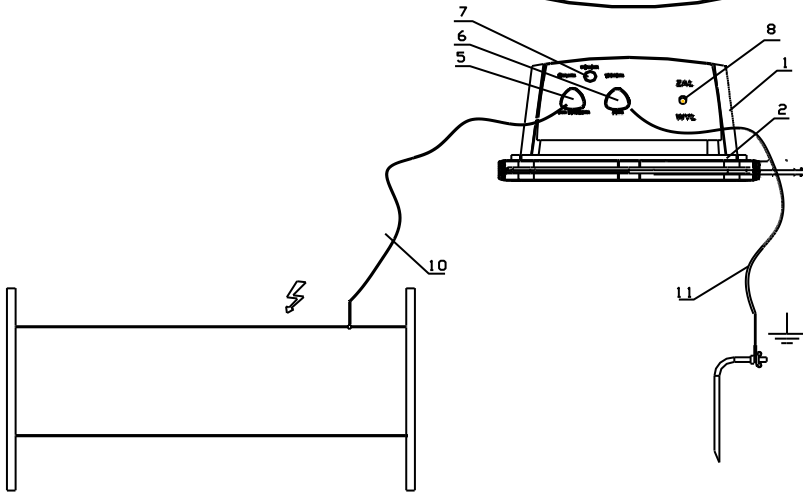
Rys. 2 Części składowe i sposób podłączenia elektryzatora EBS-872/M do zasilacza AC 12V/1000mA, linii ogrodzenia /Lo/ i linii uziemienia /Lu/
