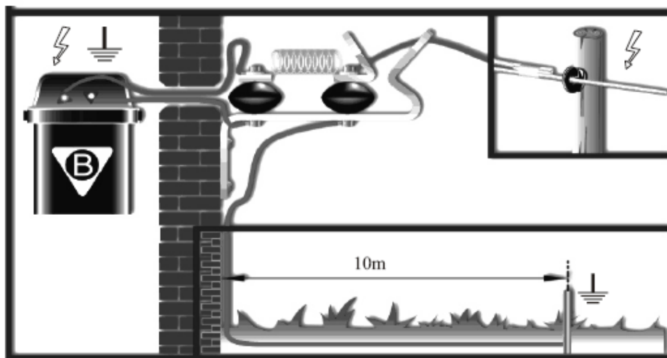
Rys. 7 Sposób przyłączenia odgromnika
