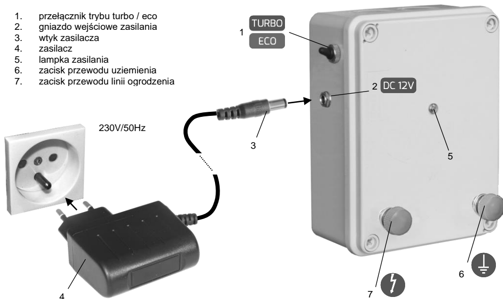
Rys. 1. Opis elektryzatora i sposób podłączenia zasilania z sieci elektrycznej ~230V
